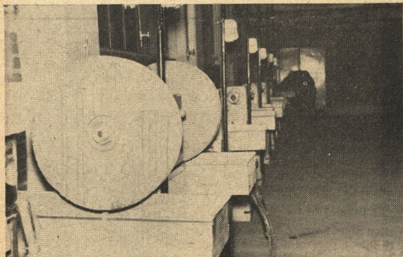
Stroji za poliranje obeskova za razsvetljavo v novem obratu brusilnice
