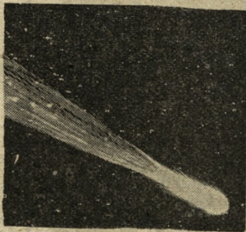
Brookov komet so opazovali astronomi leta 1911.
