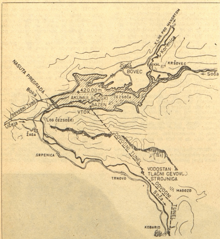
Takšna je situacija naprav HE Trnovo. Lepo je vidna oblika bodočega jezera, prav tako položaj poplavljenе Cezsoče.
