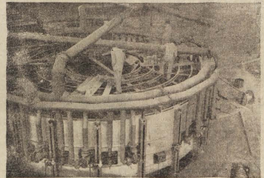
Zadnja dela pri postavljanju krožne peči v valjarni, prve te vrste v Jugoslaviji. Tu bodo segrevali ingote, iz katerih bodo potem izdelali brezšivne cevi. Peč bodo kurili z nafto ali s plinom.
