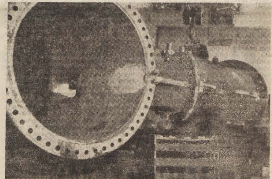
Spiralna Francisova turbina, ki jo bodo izdelali v Litostroju do konca tega leta in poslali na HC Jablanico. Turbina bo teška 150 ton in bo imela 31.000 KS. V Litostroju bodo izdelali še štiri take turbine, ki so doslej največje, kar jih je izdelal Litostroji. Končno je to ena največjih turbin na Balkanu. Glavni projektant je bil inženir Kasović. Izdelala pa sta načrte tehnik Slavko Urbančič ter Erik Mihevc. Na sliki vidite ohišje spiralne turbine z dva metra velikim vstopom v spiralo.
