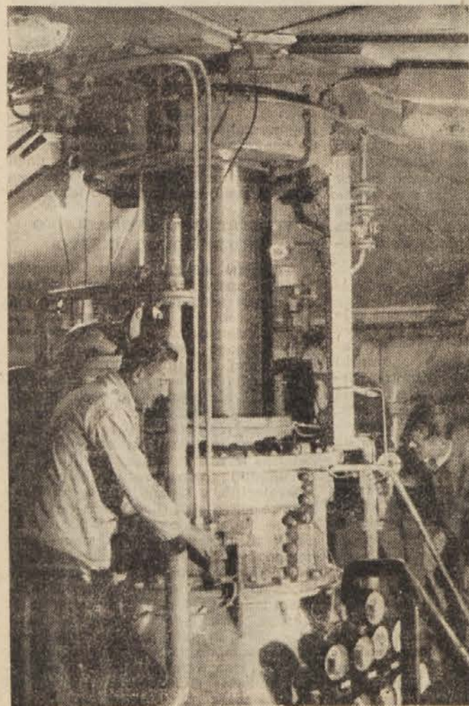
Pri turbini na hidrocentrali Mariborski otok
