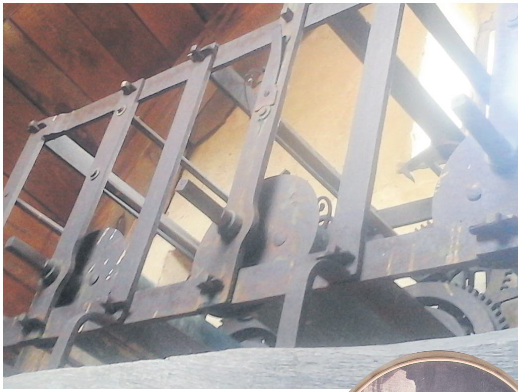
Ura v Podčetrtku ima mehanizem William Clement. Po Kukovičičevih besedah je edini ohranjen tovrstni mehanizem angleškega tipa še v Marezigah nad Koprrom in v muzeju zgodovine znanosti v Angliji. (Foto: Samo Kukovičič)
