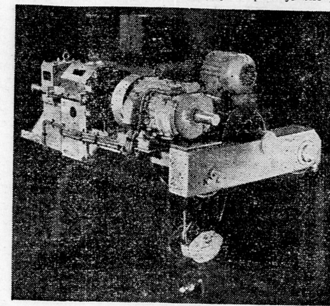
Lahki maček »lama« nosilnosti 5 ton
