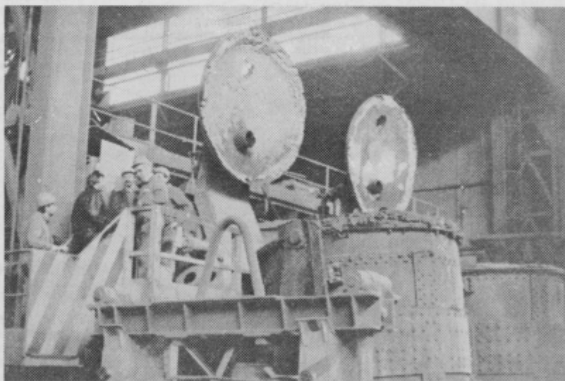
Na fotografiji sta dva livarska lonca. Desni je normalno visok, levi pa je za 252 milimetrov nadgrajen usodni lonce številka 3, ki se je prevrnil v soboto zjutraj. S tem, ko so ga nadgradili in ga preveč napolnili, se mu je spremenilo težišče.
