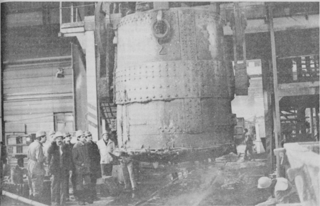
Huda nesreča, ki se je pripetila v soboto zjutraj nekaj minut pred peto uro v jeklarni 2 v štorski železarni je zahtevala pet življenj, dva huje ranjena delavca pa so odpeljali v bolnišnico. Na fotografiji je ponovca številka 3, ki se je prevrnila, iz nje pa je pljusnilo 50 ton raztaljenega jekla s temperaturo 1600 stopinj Celzija. Ponovco so nadgradili za 252 milimetrov, jo preveč napolnili, neizpravna pa so bila tudi varovala, ki skrbijo, da se ponovca ne prevrne. Foto: S. ŠROT
