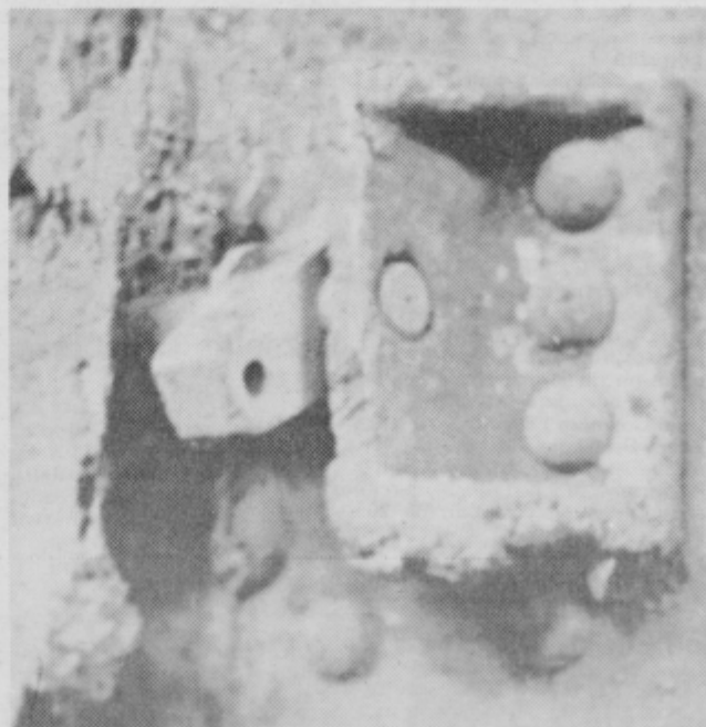
Varovalka, ki preprečuje nagib lonca; eno od varovalk je ponovčar kar odvaril (ker je bila zalita s talino), druge pa tudi niso dosegle položaja, v katerem bi lahko preprečile nagib lonca.
