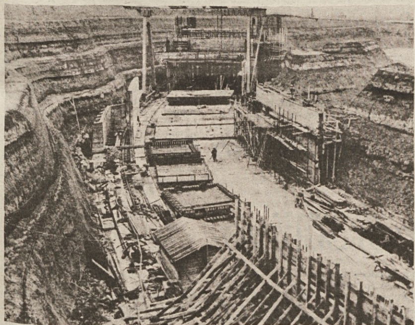
Gradnja protonskega sinhrotrona leta 1967 v Ženevi. Preden je bila izbrana ta lokacija, je obstajala možnost, da bi ga Evropska organizacija za jedrsko raziskovanje (CERN) gradila pri Doberdobu
