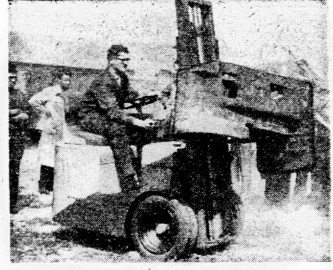
Tovarna »Indos« v Ljubljani je izdelala vilniški nakladalec z nosilnostjo 1000 kg. Hidravlično dvigalo tega stroja dvigne tovora do višine dva metra in pol in je prvi izdelek te vrste v naši državi. Nakladalec bo razstavljen na zagrebškem velesejmu.
