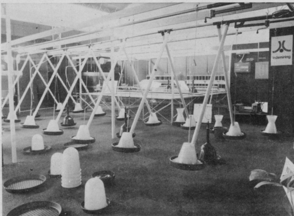
Na posnetku je vidna oprema za »viseči sistem avtomatskega hranjenja in napajanja perutnine«, v ozadju so gnezda in sedala za matično jato!
